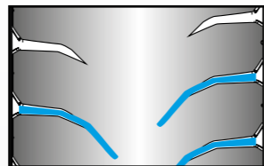
REGROOVING PATTERN 315/80 R 22.5
